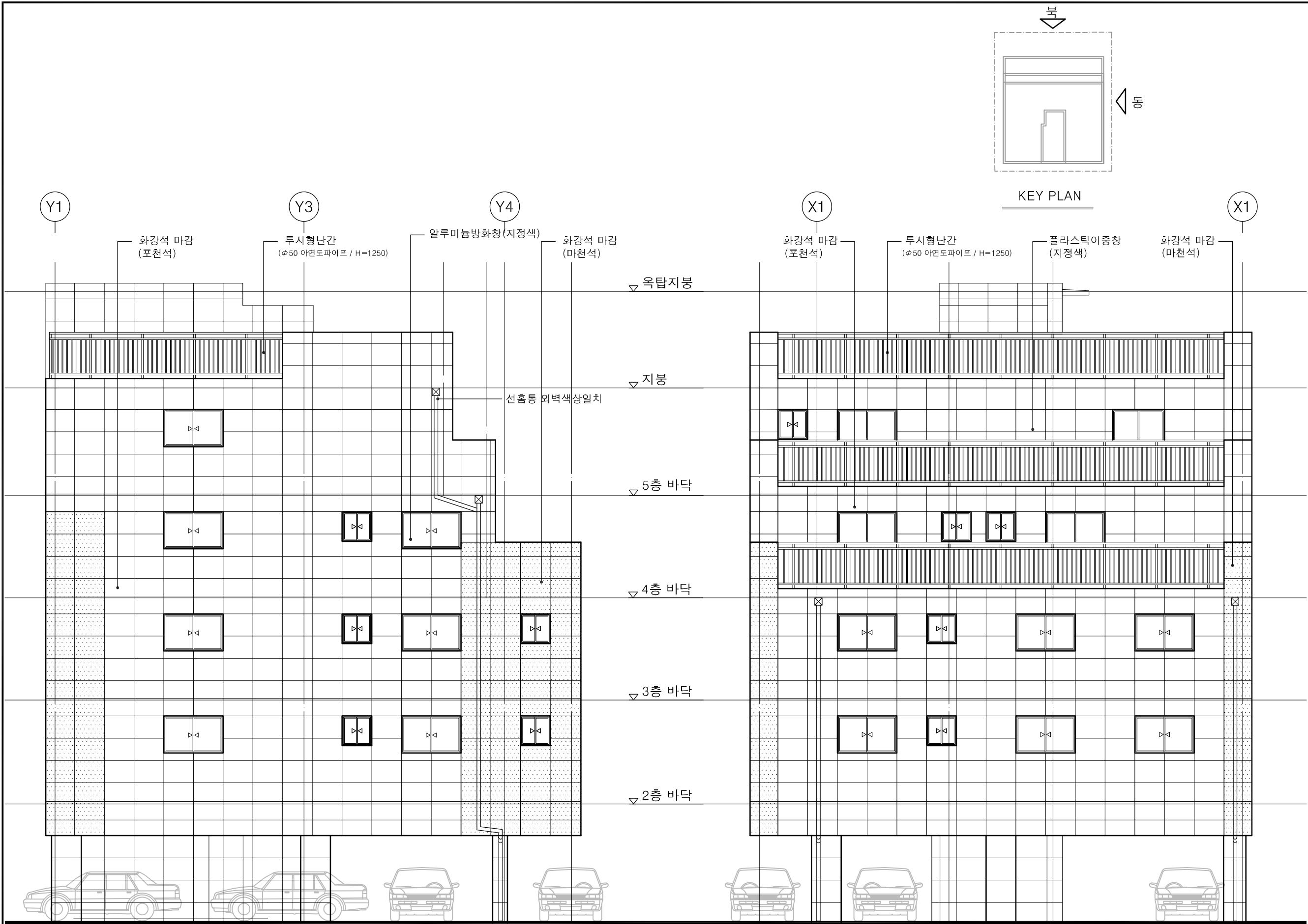
1 동측면도 축척 : 1 / 100
